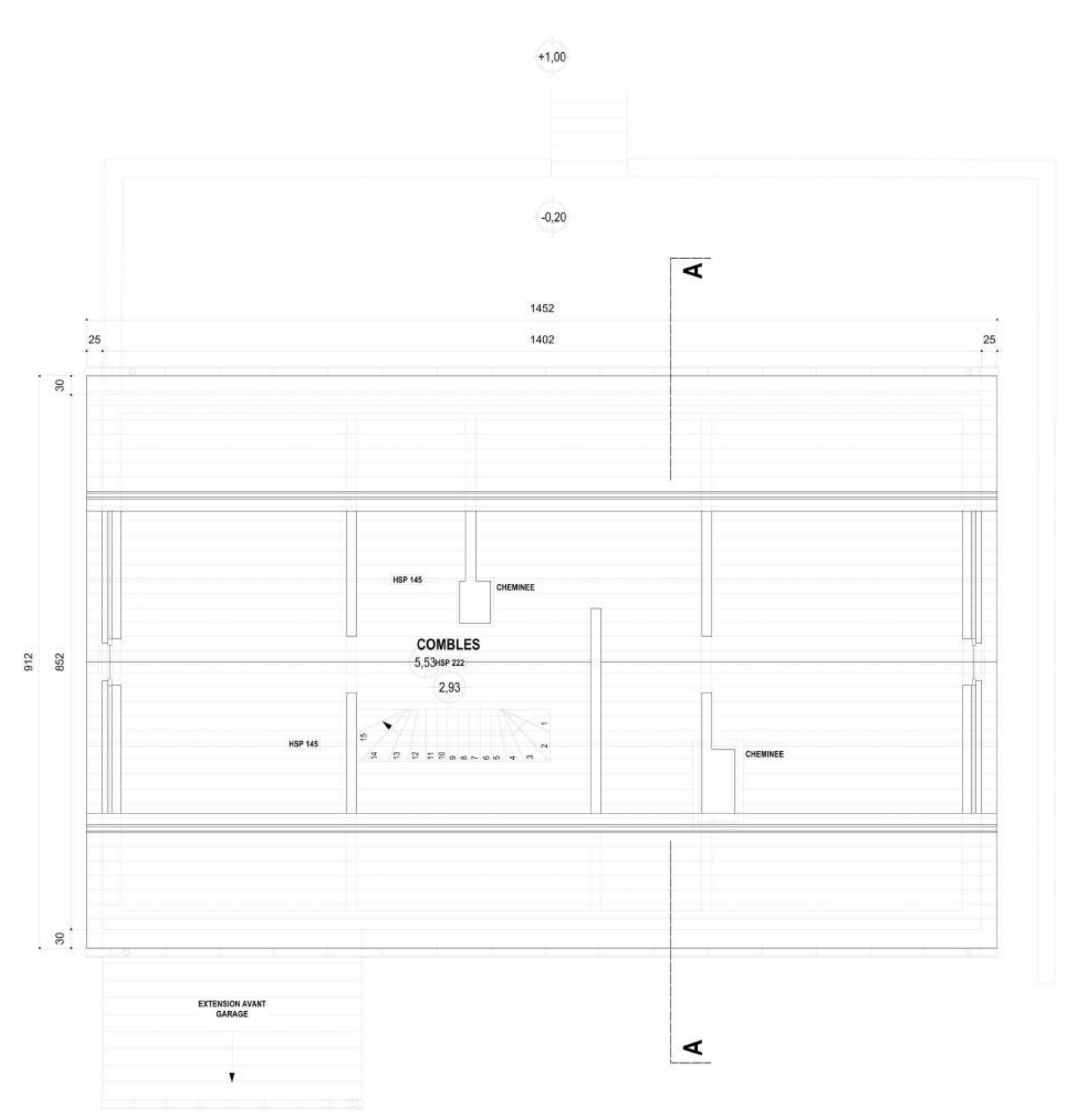
PLAN DE TOITURE
