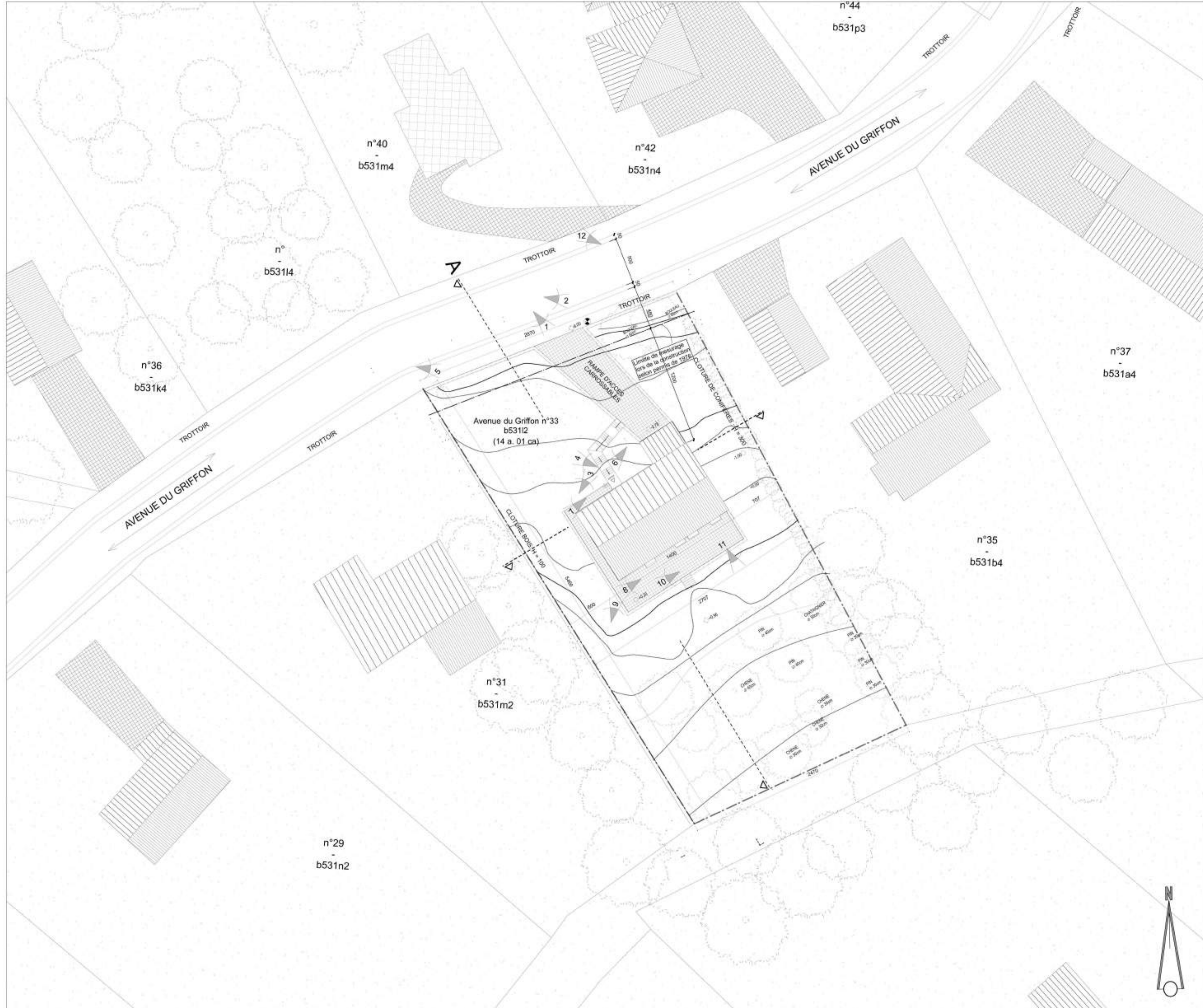
PLAN D'IMPLANTATION ech:1/250
