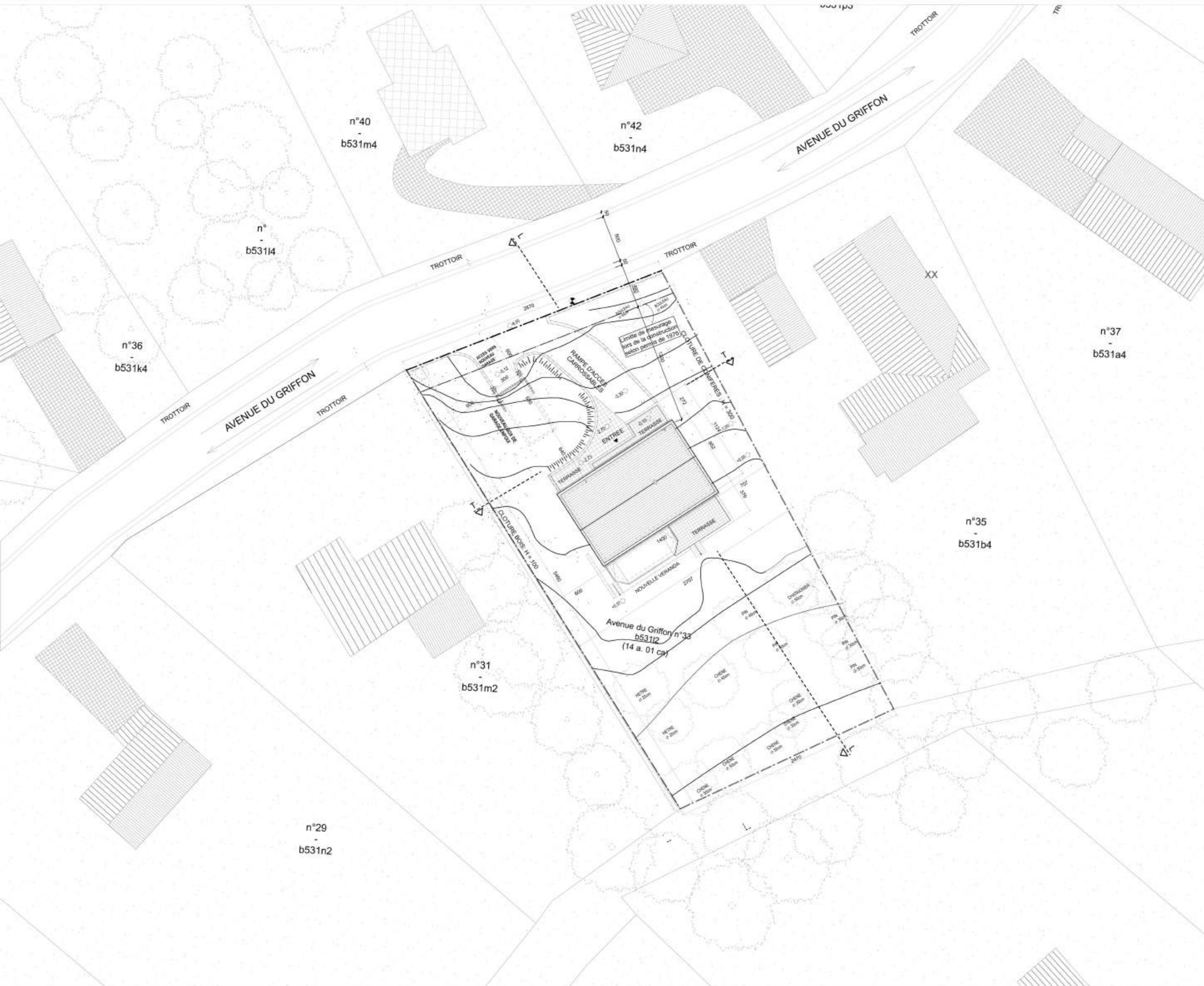
PLAN D'IMPLANTATION ech:1/250
